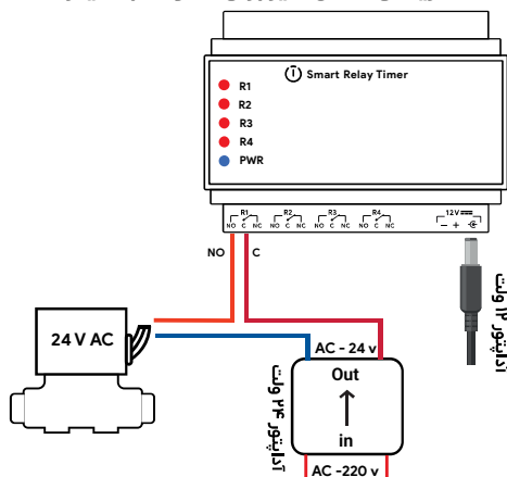
طریقه‌ی اتصال شیر برقی ۲۴ ولت به تایمر
