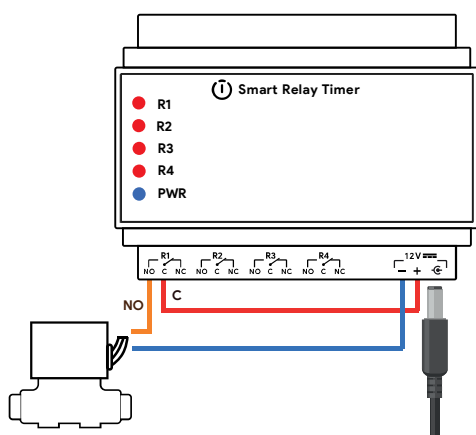
طریقه‌ی اتصال شیر برقی ۱۲ ولت به تایمر
