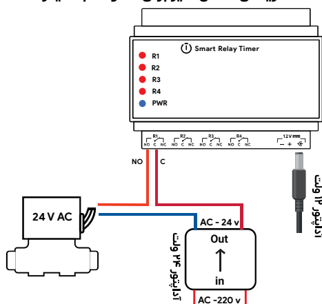
طریقه‌ی اتصال شیر برقی ۲۴ ولت به تایمر
