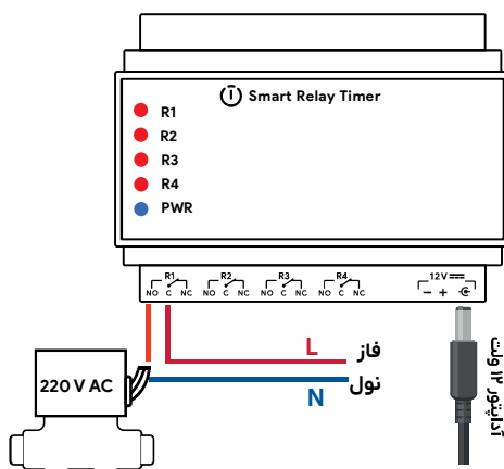
طریقه‌ی اتصال شیر برقی ۲۲۰ ولت
