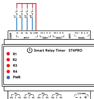
نحوه اتصال سوییچ به ورودی تایمر
