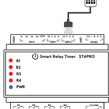
نحوه اتصال سنسور دما و رطوبت
