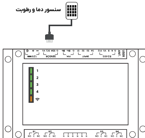
نحوه اتصال سنسور دما و رطوبت
